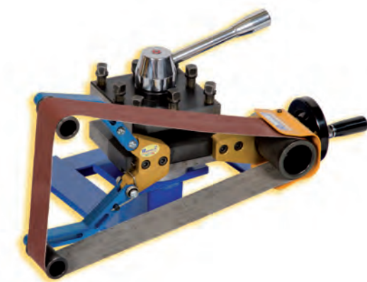
DISPOSITIVO SMERIGLIATORE PER TORNI
